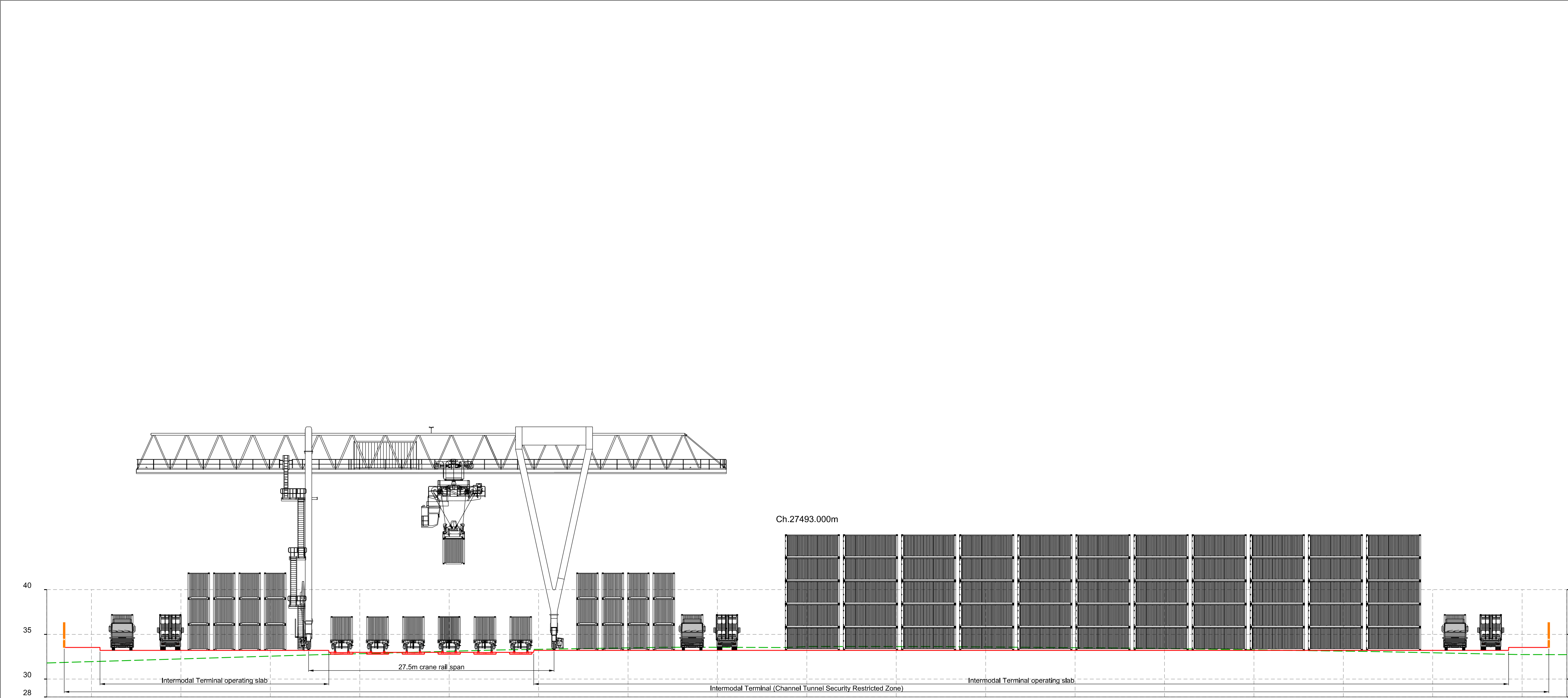
SECTION G SCALE: H 1:250, V 1:250. DATUM: 28.000
